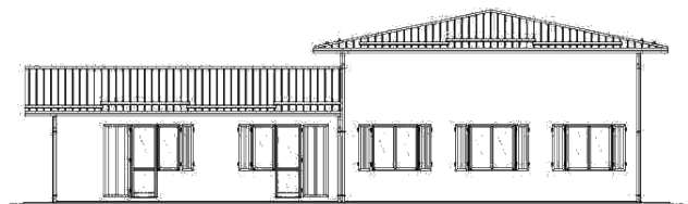
PROSPETTO EST
